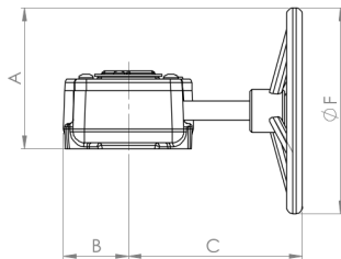
Handhebel DN125- DN200 aus Stahl
