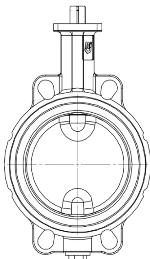
DN80-150
