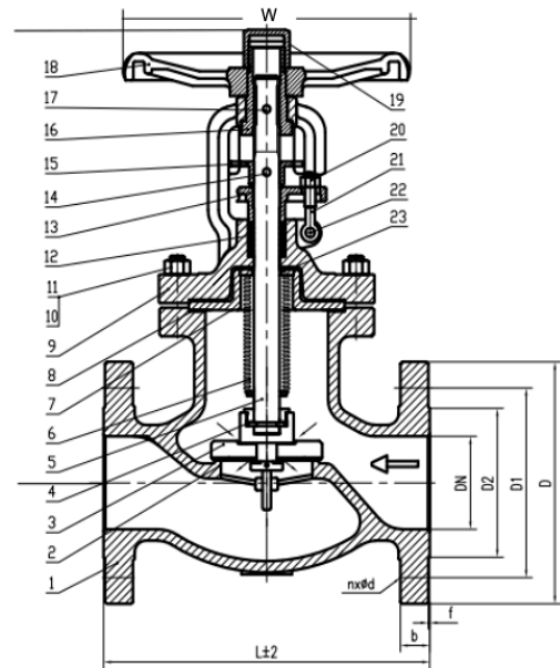
Abbildung gilt bei AV05: PN16 von DN125 bis DN250 PN40 von DN125 bis DN250
