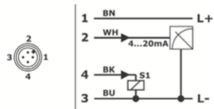
4-Leiter – Ausgang 1x Schalter PNP / 1x Strom 4 - 20mA
