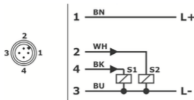
4-Leiter – Ausgang 2x Schalter PNP
