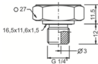
G 1/4" ISO 228-1
