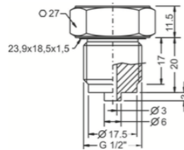
G 1/2" ISO 228-1 - DIN 837-3
