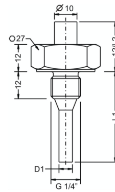
G 1/4"
