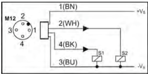
2x PNP
