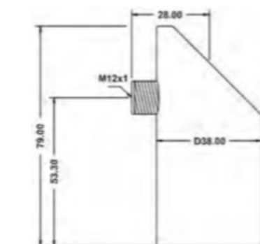
Boîtier de raccordement
