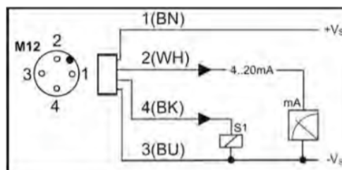
1x PNP, 1X analogique
