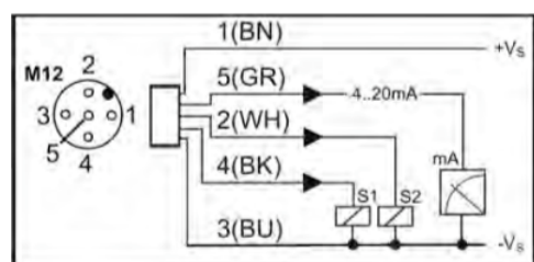
2x PNP, 1x analogique
