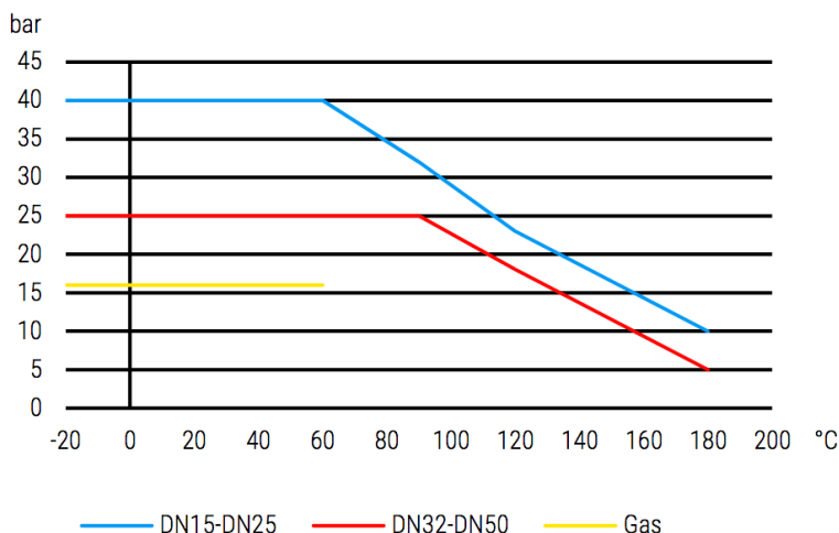
Diagramme pression-température
