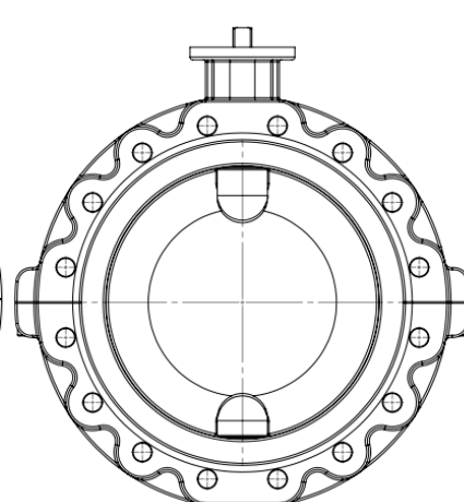
DN350 jusqu'à DN600 PN10-16 et ANSI 150
