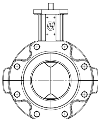
DN100 jusqu'à DN200 – ANSI 150 DN80 jusqu'à DN150 – PN10-16
