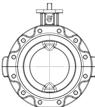
DN250 jusqu'à DN300 – ANSI 150 DN200 jusqu'à DN300 – PN10
