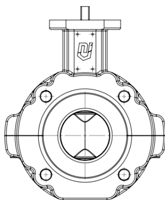
DN65 jusqu'à DN80 ANSI 150
