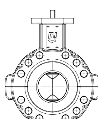
DN65 PN10-16
