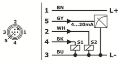
Uscita a 5 fili 2x interruttore PNP / 1x corrente 4 – 20 mA
