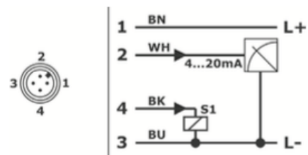
Uscita a 4 fili – 1x interruttore PNP / 1X corrente 4 – 20 mA
