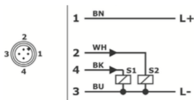
Uscita a 4 fili 2x interruttore PNP
