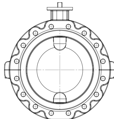
DN350 - DN600
