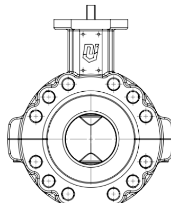
DN65 PN10-16
