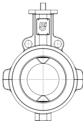
DN50 - DN100
