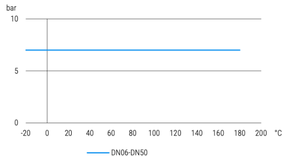
Druck-Temperatur-Diagramm pressure-temperature-diagram
