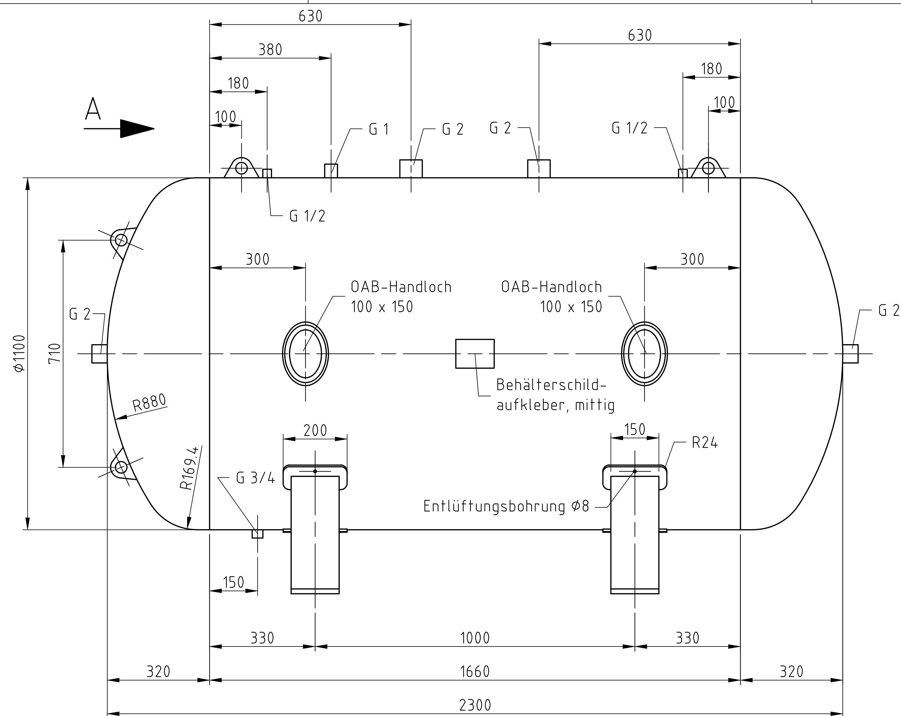
Ansicht A
