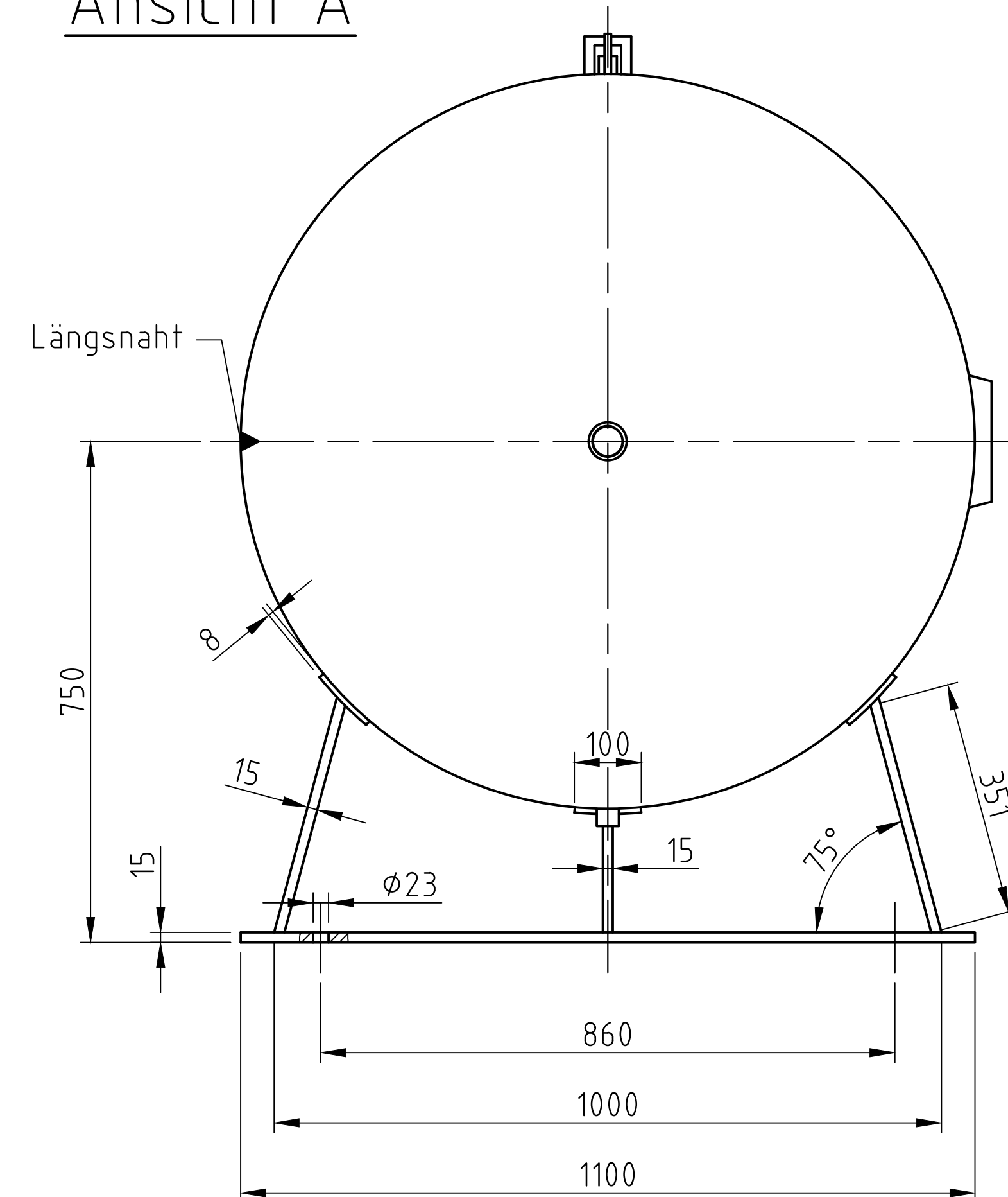
Ansicht A
